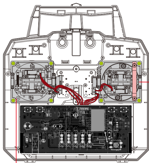
右总成座 right seat assembly
